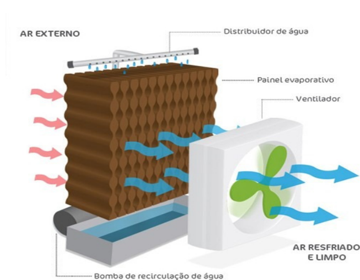
Figura 1 – Funcionamento ilustrativo do climatizador evaporativo.
